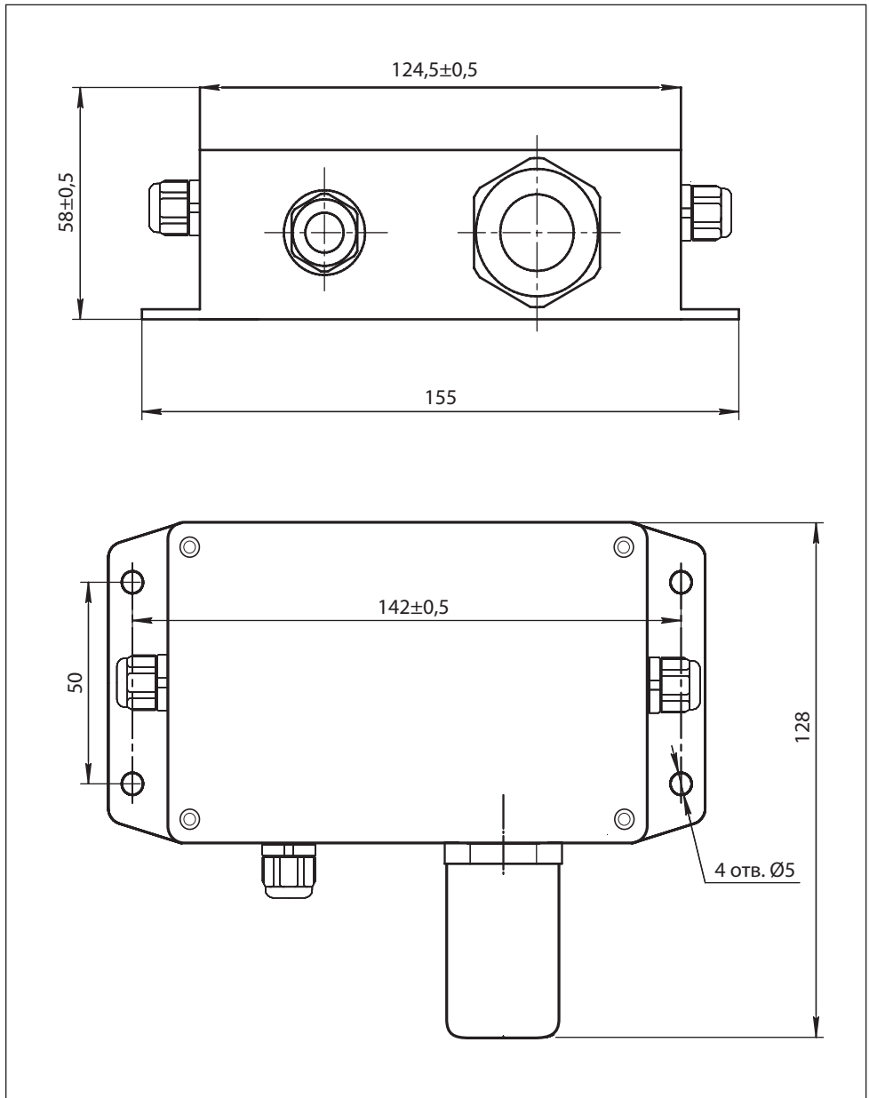
Рис.5. Габаритный чертеж газоанализатора "Сенсон-СД-7033"
