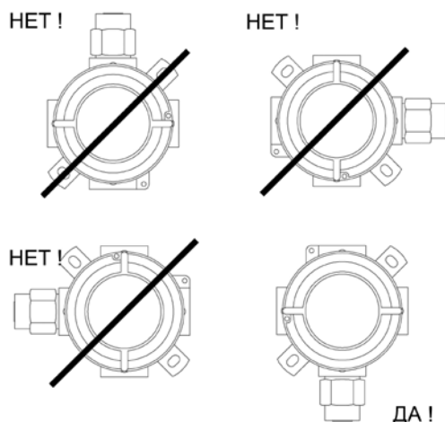
Рис. 3: Правильная установка
