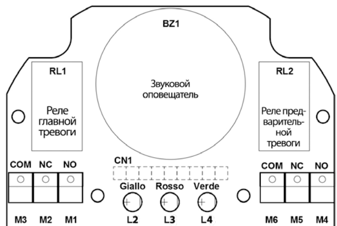
Рис. 4: Вид прибора изнутри (плата вывода)
