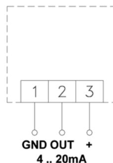
Рис. 5: Электрическое подсоединение
